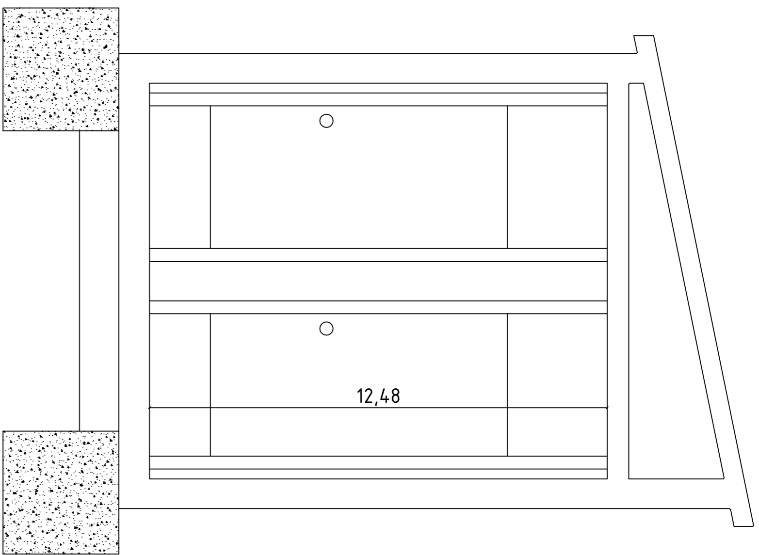
SECCIÓN TRANSVERSAL A-A'
